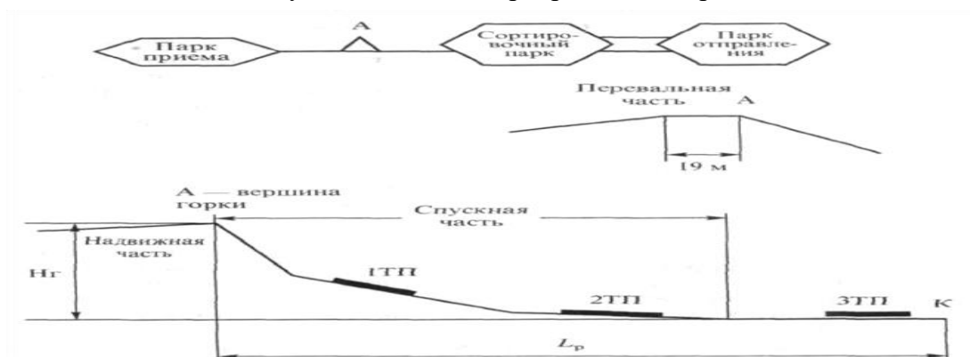
Рисунок 2 - Схема сортировочной горки
