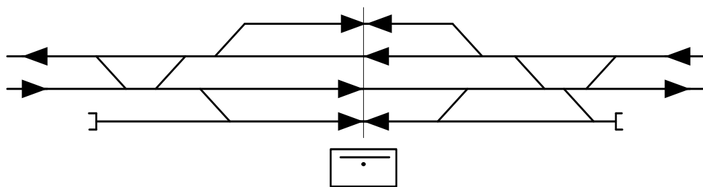
Рисунок 3.1- Макет схематического плана станции
