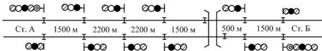
Рисунок 1- Путьевой план перегона
