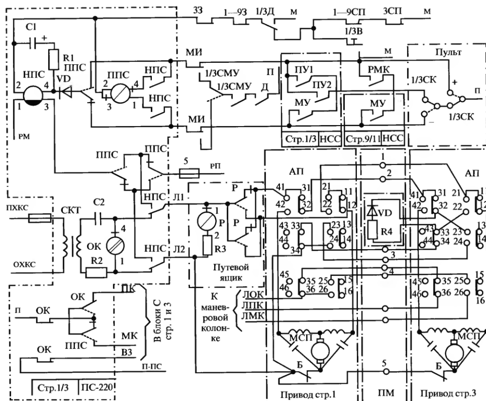
Рисунок 1 - Двухпроводная схема управления спаренной стрелкой
