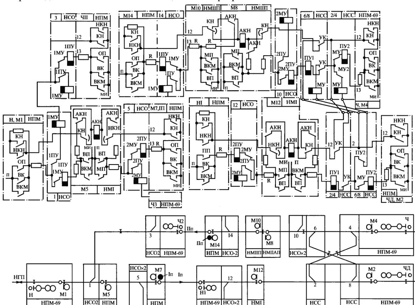
Рисунок 1- Схема автоматических кнопочных и управляющих стрелочных реле
