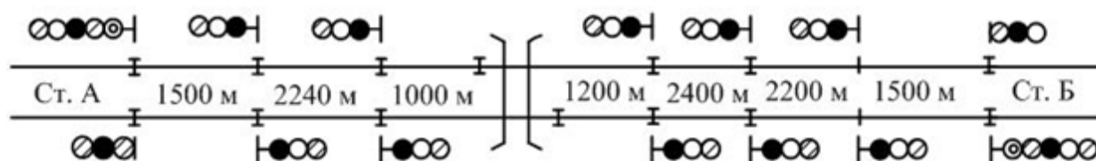
Рисунок 1- Путевой план перегона
