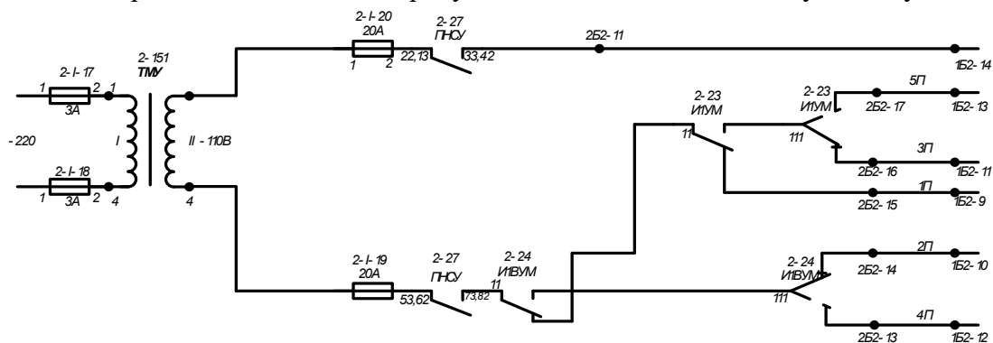
Рисунок 3.1 - Принципиальная схема
