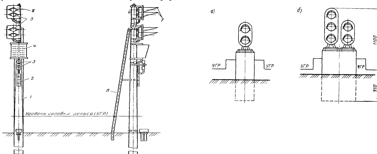
Рисунок 3.1 - Железнодорожные светофоры.
