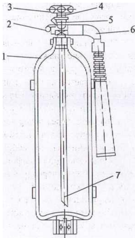
Рис. 1. Углекислотный Температурный режим хранения и применения огнетушитель ОУ-5 1 -углекислотных огнетушителей от -40^{\circ}\text{C} до +50^{\circ}\text{C} .
