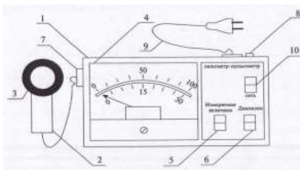
Рис. 2. Внешний вид люксметра- «БЖшМ»
