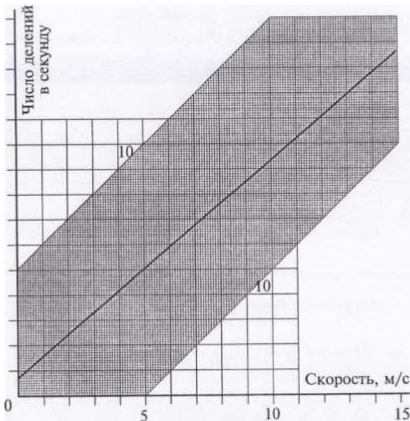
График анемометра
