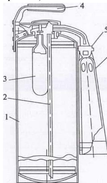
Рис. 1. Воздушно-пенный огнетушитель ОВП-Ю.
