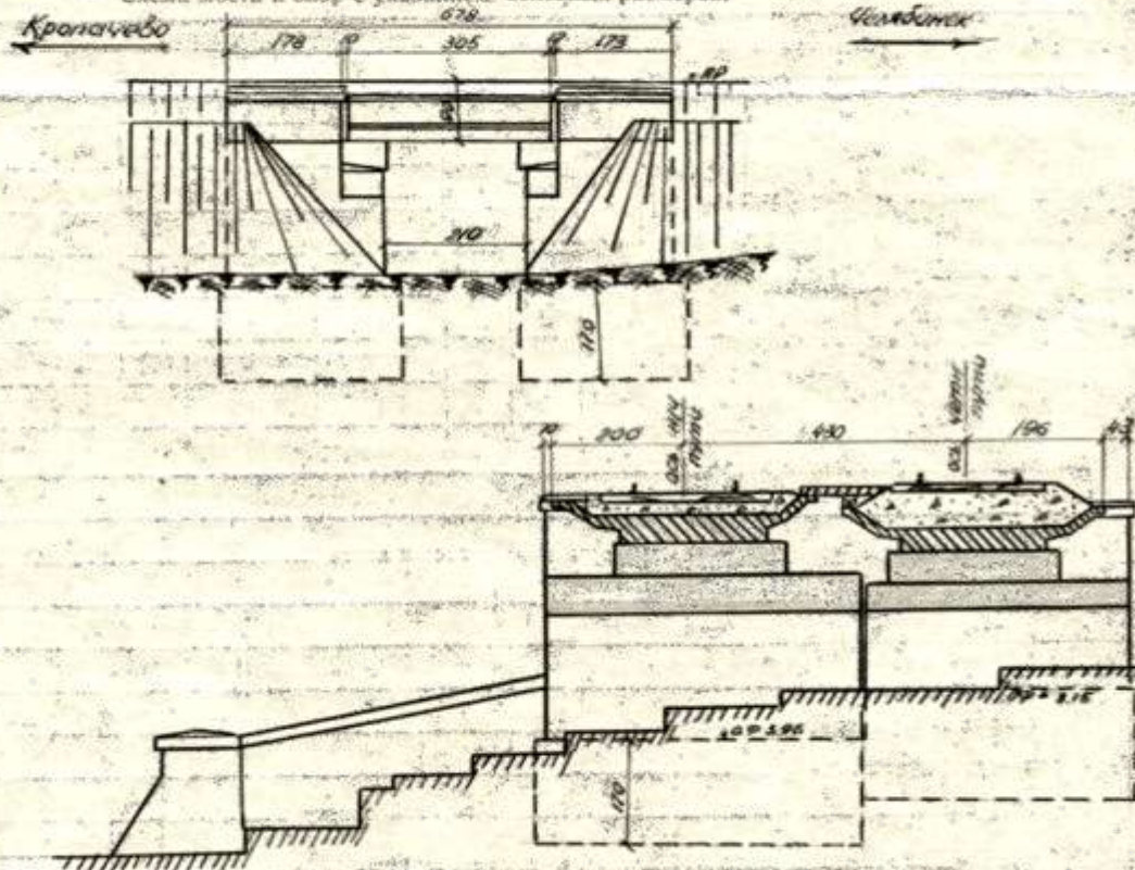
Схема моста и опор с указанием основных размеров:
