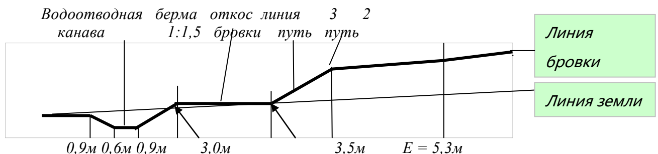
Рисунок 6 Часть поперечного профиля
