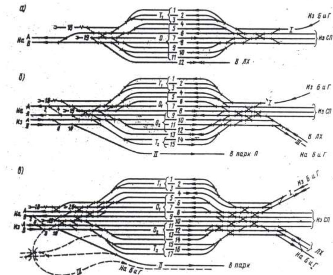
Рис 2 Схемы транзитно-отправочного парка односторонних сортировочных станций
