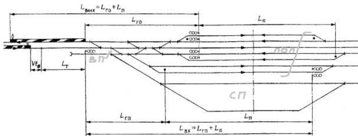
Рисунок 1 Типовая схема для расчета числа путей в соответствии с индивидуальным заданием:
