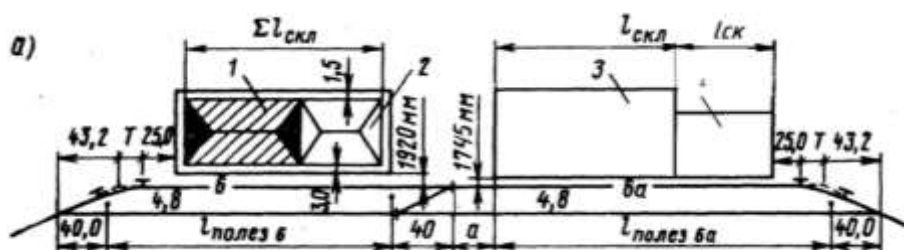
Рисунок 9 Схема размещения грузовых устройств на неопорной промежуточной станции: 1-крытый склад, 2-крытая платформа, 3- контейнерная площадка, 4- навалочная площадка Т – тангенс закрестовинной кривой (м) (из ПР №4),
