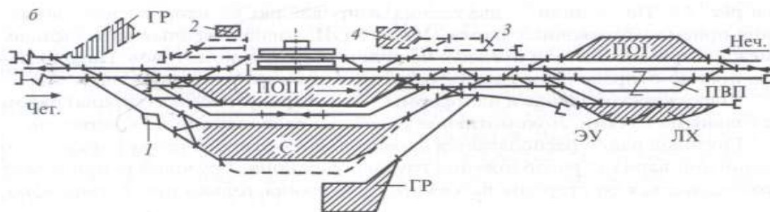
Рисунок 1 Схема участковой станции однопутной линии продольного типа: 1 – горка малой мощности, 2 – багажные устройства, 3 – пути стоянки пассажирских составов, 4 – вариант размещения устройств на станции.
