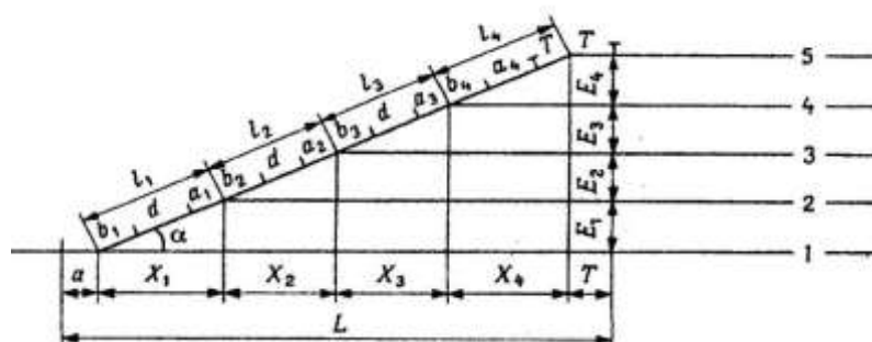
Рисунок 3 Стрелочные улицы под углом крестовины.
