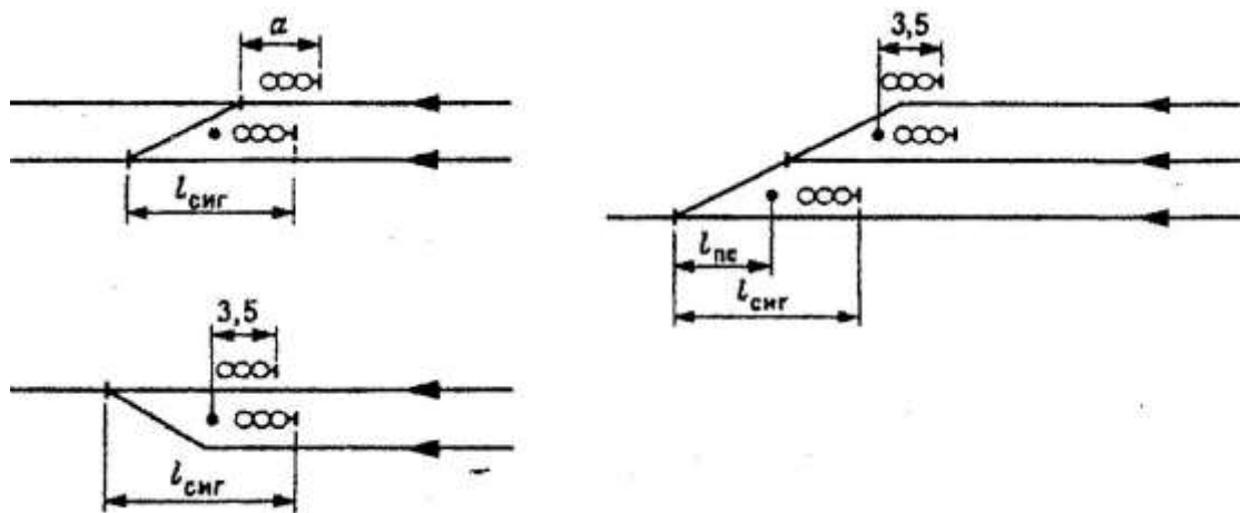
Рисунок 3 Установка выходных светофоров
