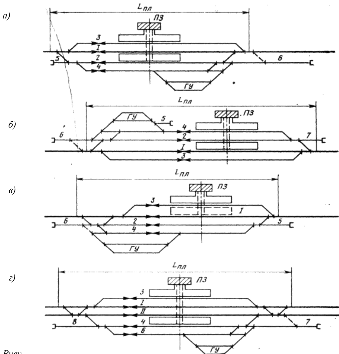
Рисунок 12 Схемы промежуточных станций с поперечным расположением путей:
