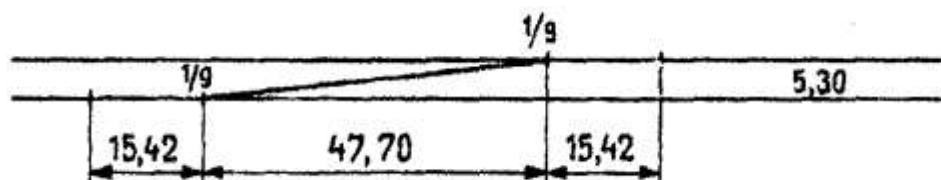
Рисунок 6 Образец выполнения сезда в масштабе 1:2000
