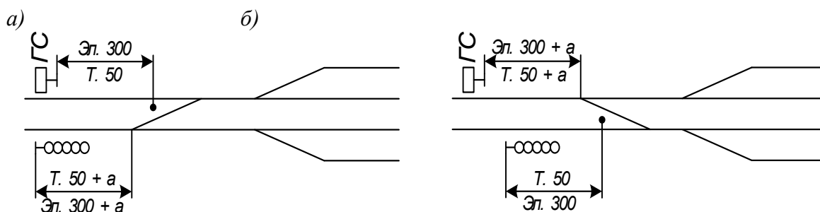
Рисунок 2 Установка входных светофоров:
