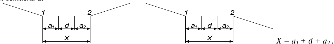
Рисунок 4 Схемы взаимного расположения стрелочных переводов при встречной укладке.
