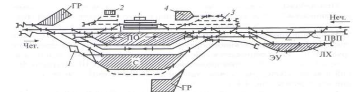
Рисунок 2 Схема участковой станции однопутной линии поперечного типа
