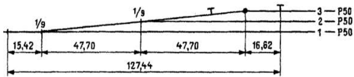
Рисунок 7 Образец выполнения стрелочной улицы под углом крестовины в масштабе 1:2000
