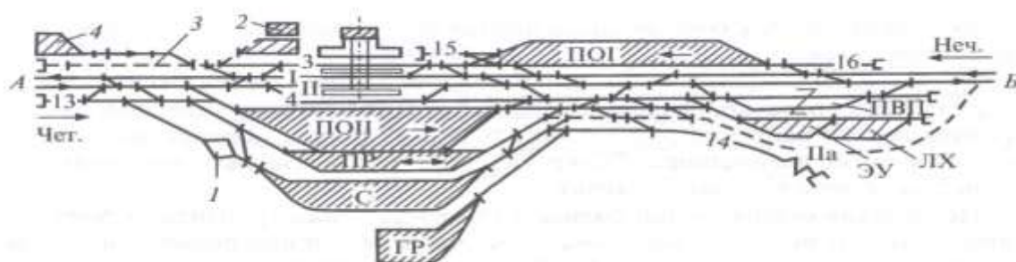
Рисунок 4 Схема участковой станции двухпутной линии продольного типа
