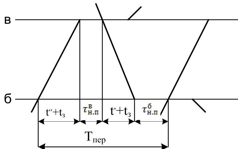
Схема 1 - поезда следуют на труднейший перегон сходу;
