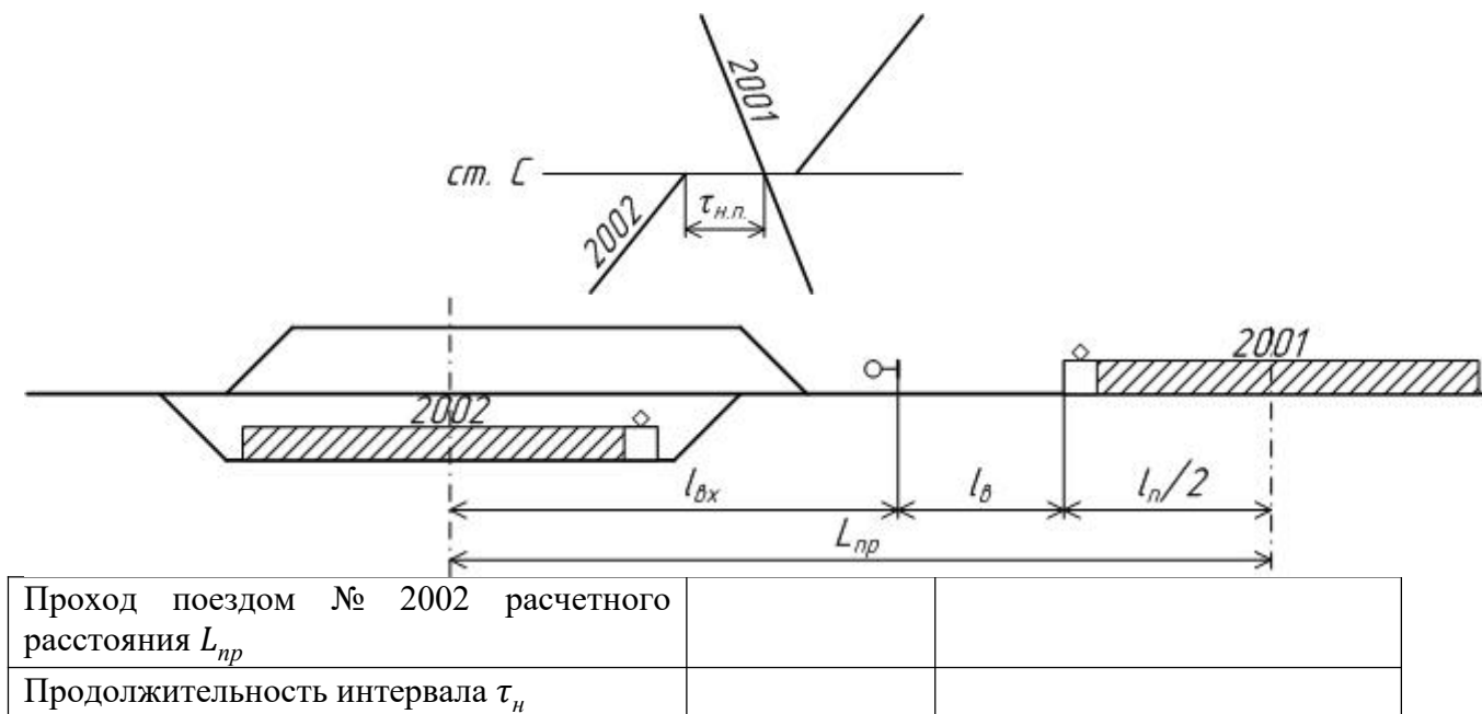
Рисунок 2 График операций при расчете интервала неодновременного прибытия при автоматической блокировке
