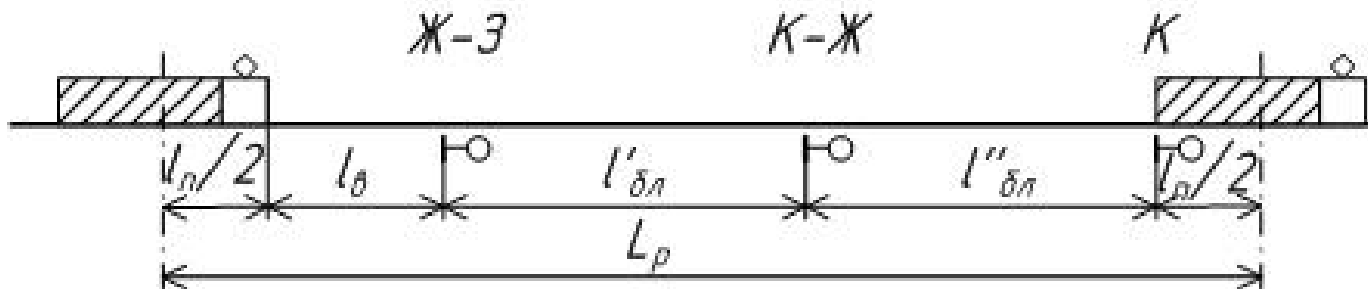
Рисунок 2 Разграничение поездов двумя блок-участками
