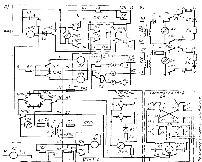
Рисунок 1- Двухпроводная схема управления стрелкой
