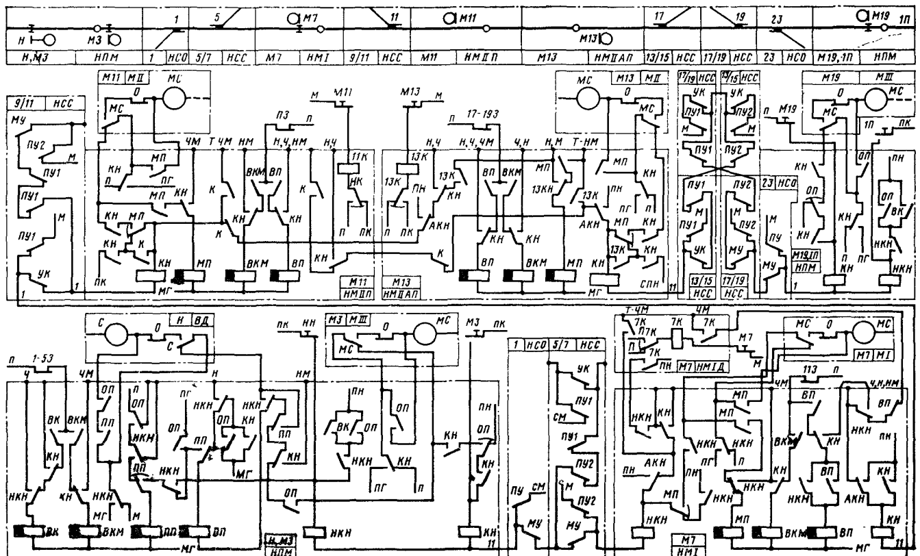
Рисунок 1 - Схема кнопочных противоповторных и вспомогательных реле.
