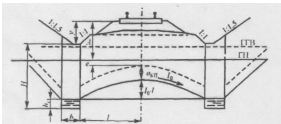
Рис.3.2 Схема двустороннего подкюветного дренажа, «ГВБ» - уровень грунтовых вод до устройства дренажа, «ГП» - глубина промерзания земляного полотна.
