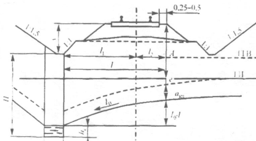
Рис. 3.1 Схема одностороннего подкюветного дренажа
