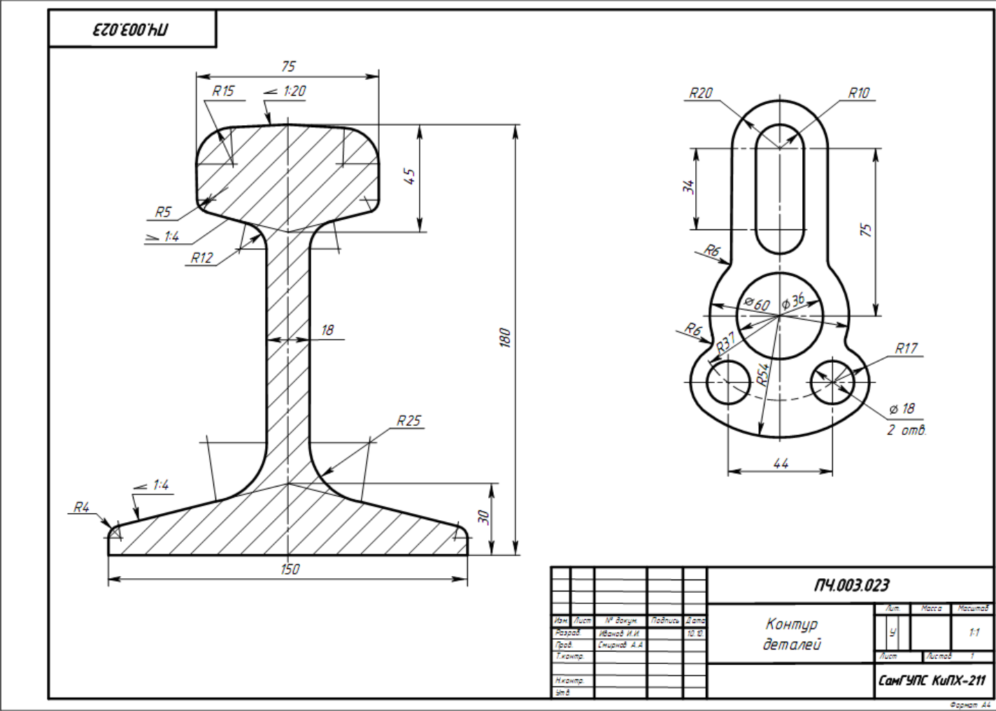
Рисунок 5 Образец выполнения задания «Контур деталей»
