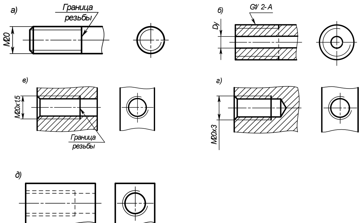
Рисунок 4 Изображение резьбы на чертежах
