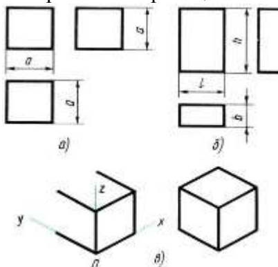
Рисунок 6 Куб и прямоугольный параллелепипед: а и б - комплексные чертежи; в- последовательность построения изометрической проекции
