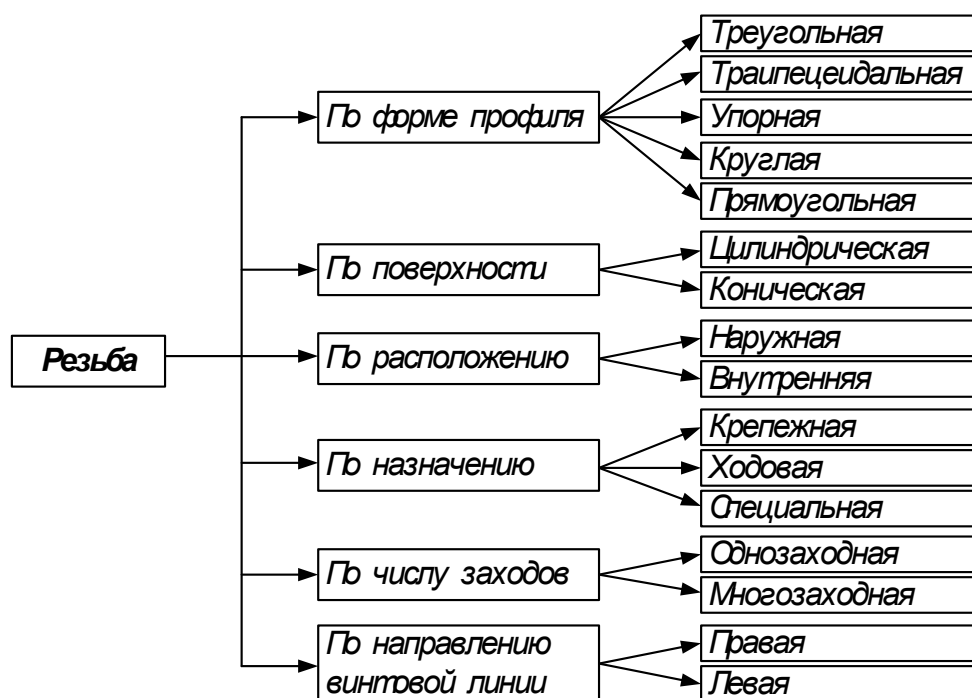
Рисунок 1 Классификация резьбы
