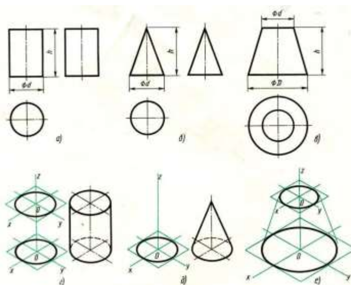
Рисунок 4 Цилиндр и конус: а, б и в – комплексные чертежи; построения изометрической проекции; г, д и е – последовательность
