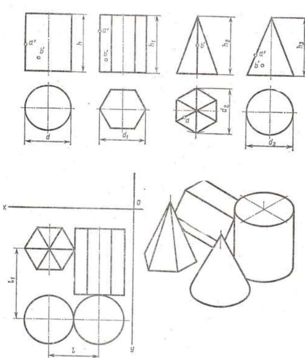
Рисунок 9 Образец задания для работы
