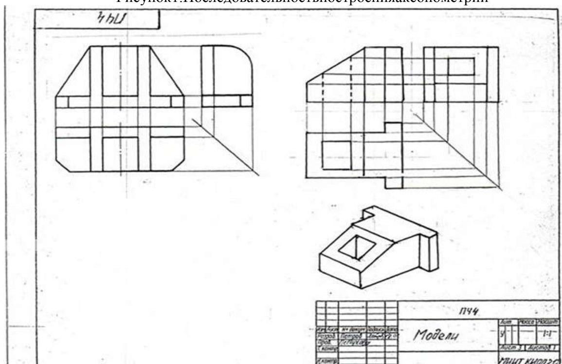
Рисунок 9 Образец выполнения задания
