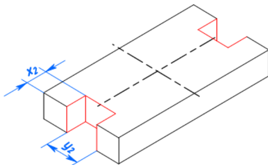
Изображение призматических пазов в основании
