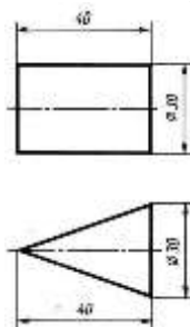
Рисунок 5 Рациональное выполнение изображений цилиндра и конуса
