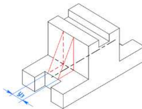
Изображение ребер жесткости
