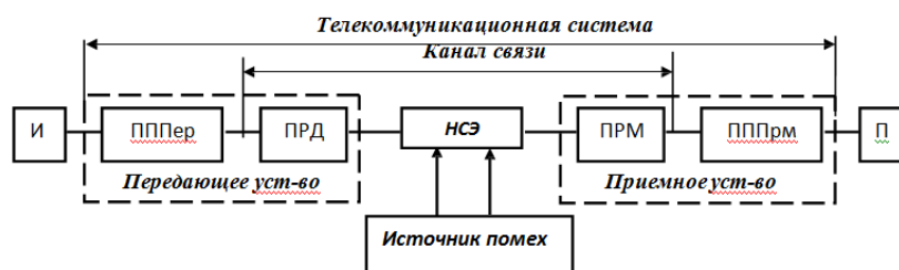
Обобщенная структурная схема систем электросвязи
