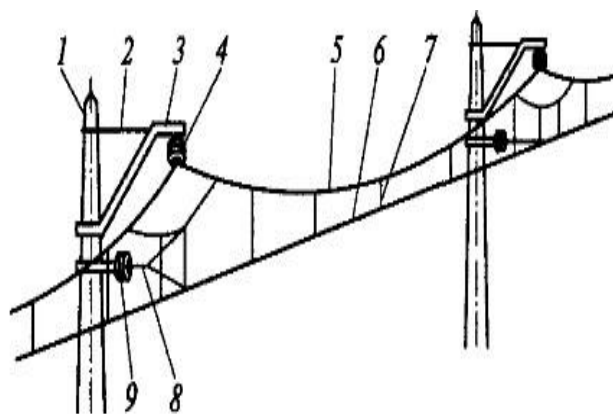
Цепная подвеска:
