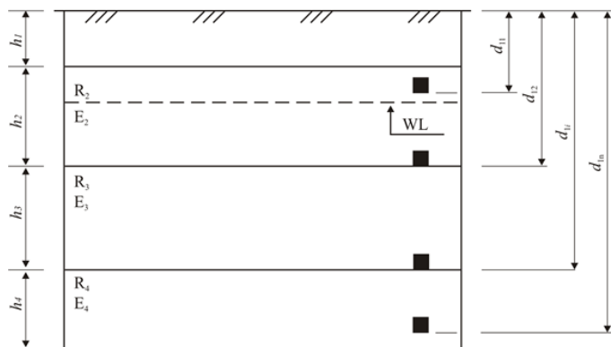
Рис. 1. Схема к определению расчетного сопротивления грунта
