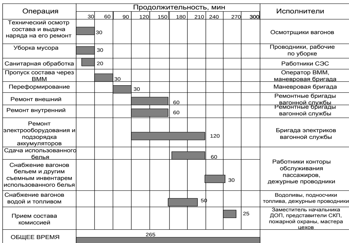
Рис. 3. График операций по обработке состава пассажирского поезда
