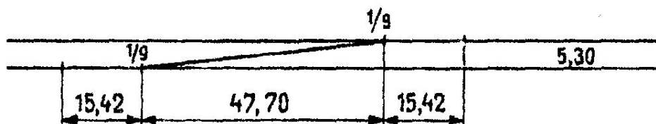
Рисунок 6 Образец выполнения съезда в масштабе 1:2000
